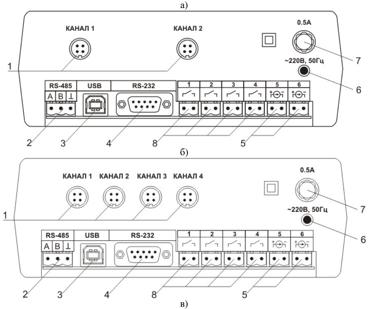
Рисунок 3.3 Вид задних панелей газоанализаторов ПКГ-4 /Х-Т-К-4Р-2А (3):
