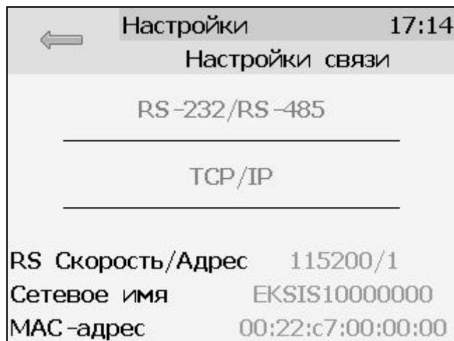
Рисунок 6.23 Экран настроек связи (ПКГ-4 /X-Т-К-4Р-2А с Ethernet)
